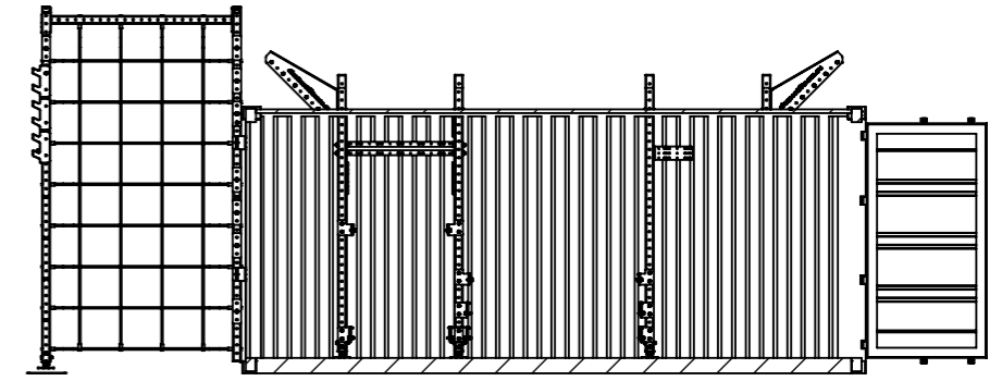
B-B 1:80
